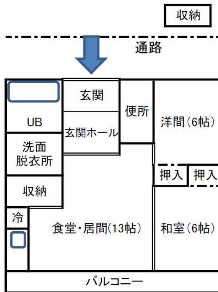
南原住宅B棟4号(2LDK) 南原住宅G棟4号(2LDK) 南原住宅 I 棟4号(2LDK)
